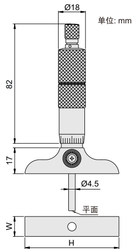
测杆(标配)
