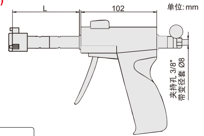
数显表(选配) 216-010-01
