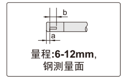
校对环规
