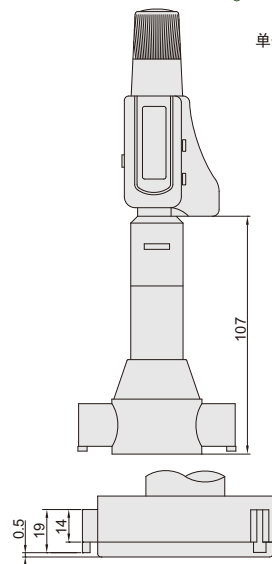
延长杆(标配)
