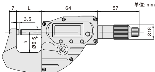
直进式测头
