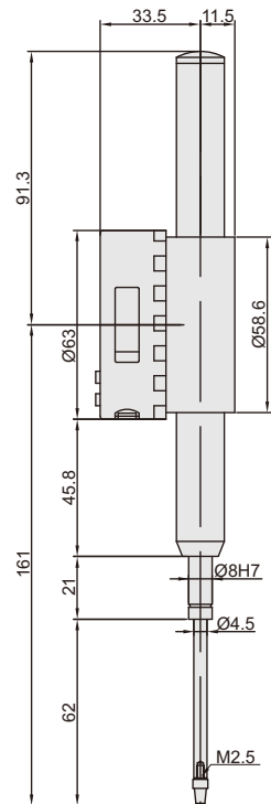
量程: 0-50.8mm
