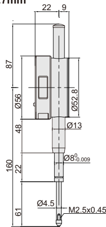
量程: 0-50.8mm
