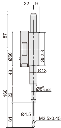
量程: 0-50.8mm
